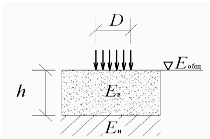
Рис. 4. Схема двухслойной конструкции:
